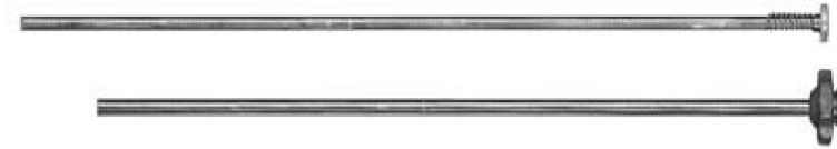
13-1630R 5 mm Schaft für zerlegbare bipolare Zange 5 mm sheath for modular bipolar forceps
