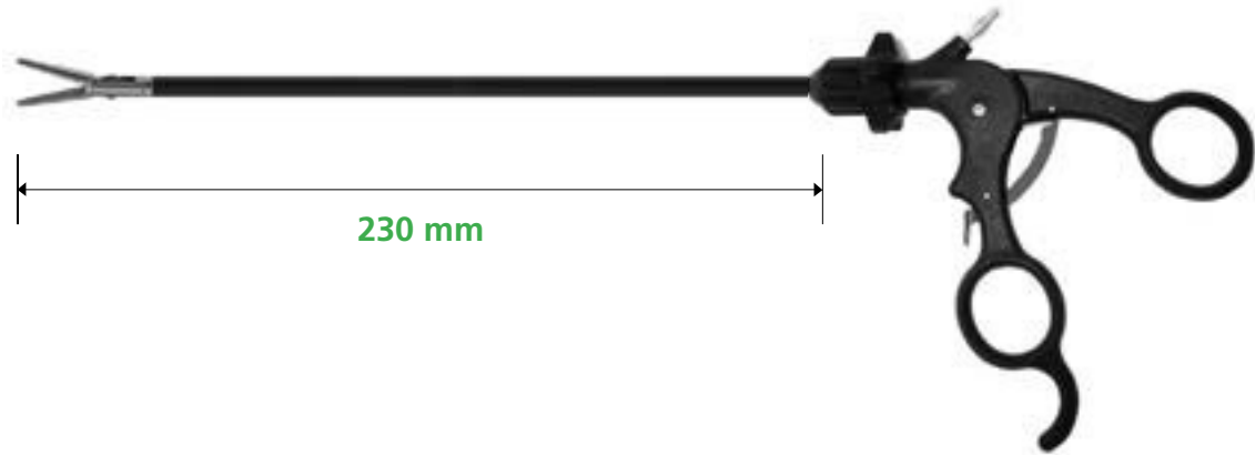
13-1601 Mikro Dissektions-Schere, 5 mm Micro dissecting scissors, 5 mm
