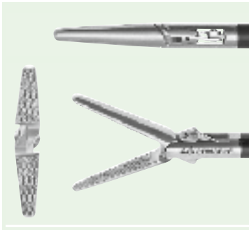
13-1604 Atraumatischer Greifer, 5 mm Atraumatic grasper, 5 mm
